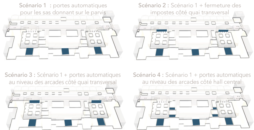
Les quatre scénarios retenus pour l'étude aéraulique
