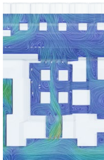
Etude aéraluque - Carte des mouvements et vitesses d'air du Hall Alsace pour une direction de vent donnée
