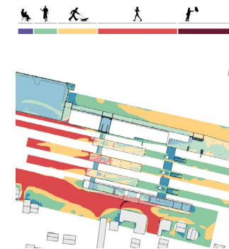
Gare de Bondy - Cartographie des niveaux de confort
