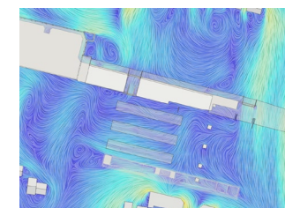
Gare de Bondy - Cartographie des vitesses de vent
